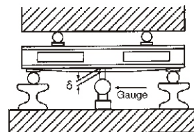
荷重測試
